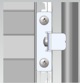
Mittelarretierung zweiteilig von 11 bis 33 mm
