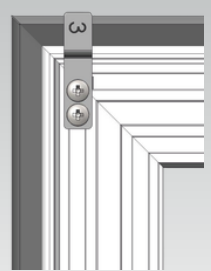
Einhängewinkel BZ3
